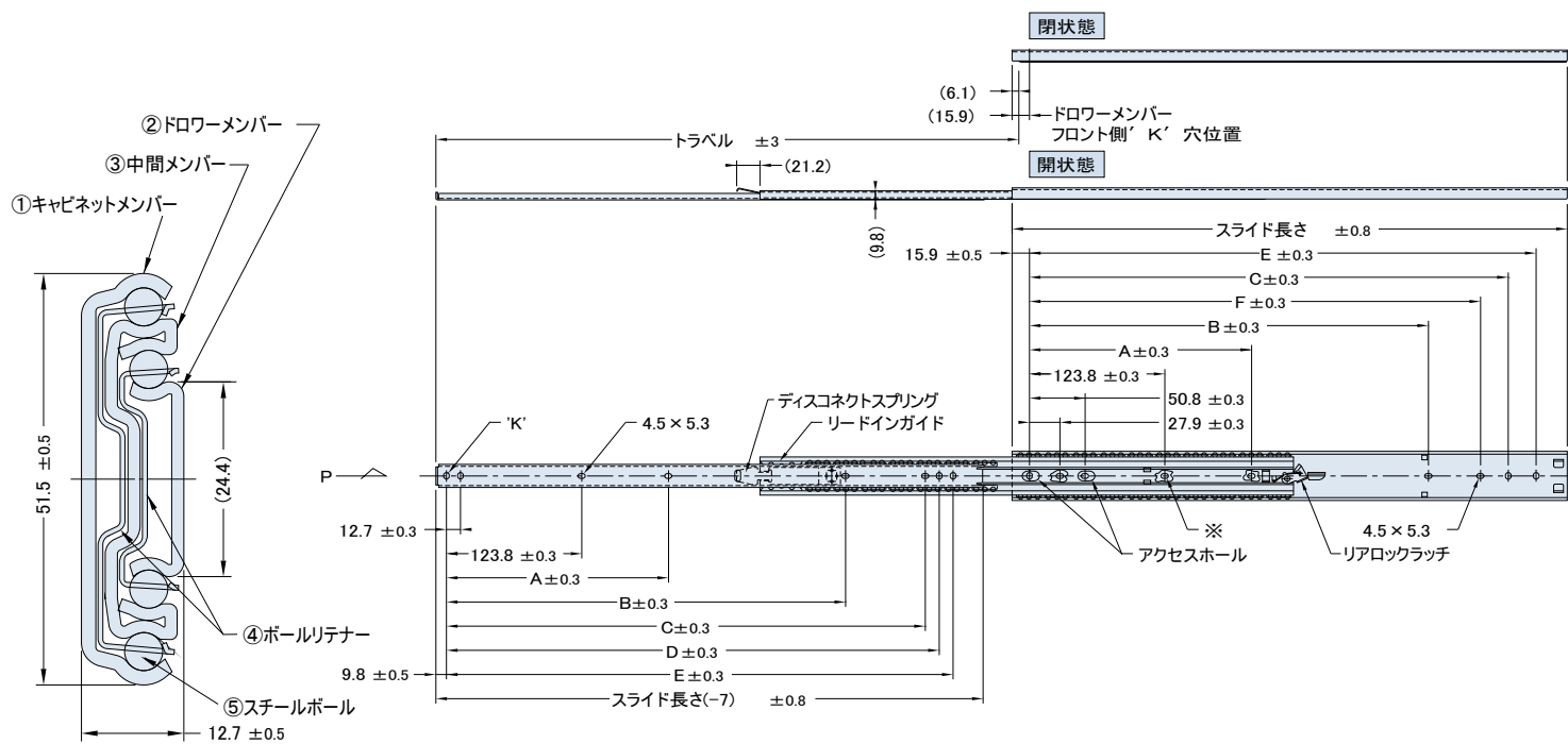
P矢視断面図 (S:1/1)
